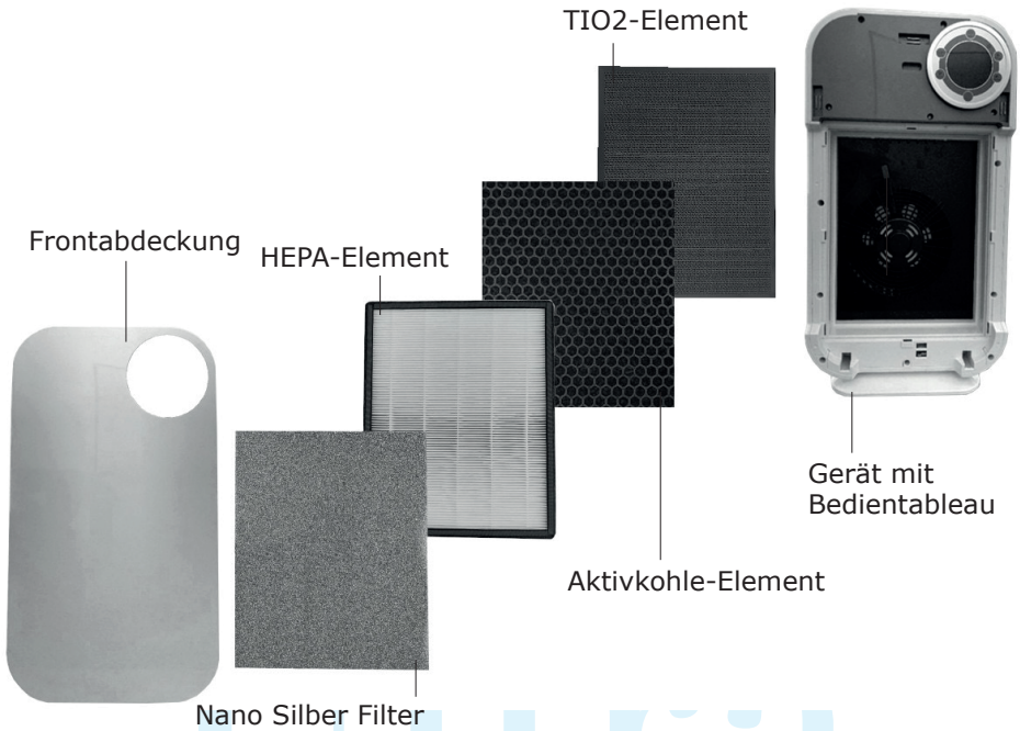
Abbildung 1 - Gerät Frontseite mit Filter
